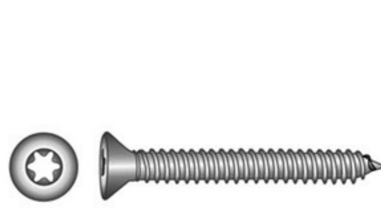
Senkkopf- Blechschraben mit Innensechsrund 14586446239
